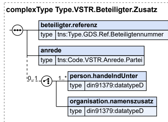
Abbildung 10.10. Type.VSTR.Beteiligter.Zusatz
