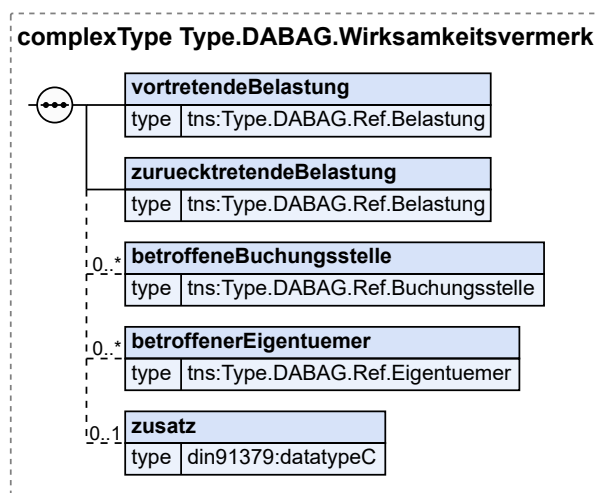
Abbildung 24.67. Type.DABAG.Wirksamkeitsvermerk
