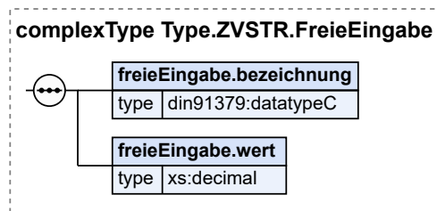
Abbildung 22.14. Type.ZVSTR.FreieEingabe
