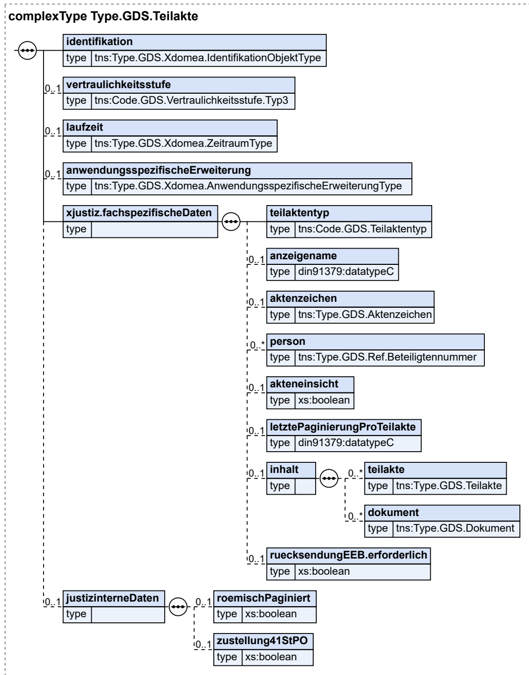
Abbildung 3.37. Type.GDS.Teilakte
