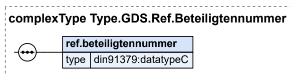
Abbildung 3.31. Type.GDS.Ref.Beteiligtenummer
