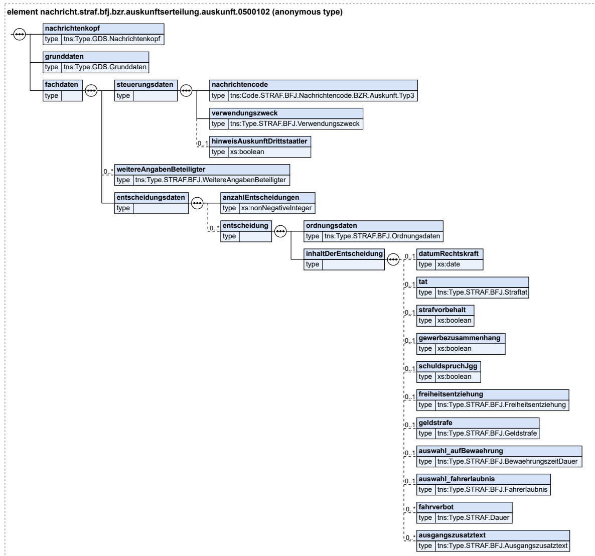
Abbildung 8.92. nachricht.straf.bfj.bzr.auskunftserteilung.auskunft.0500102
