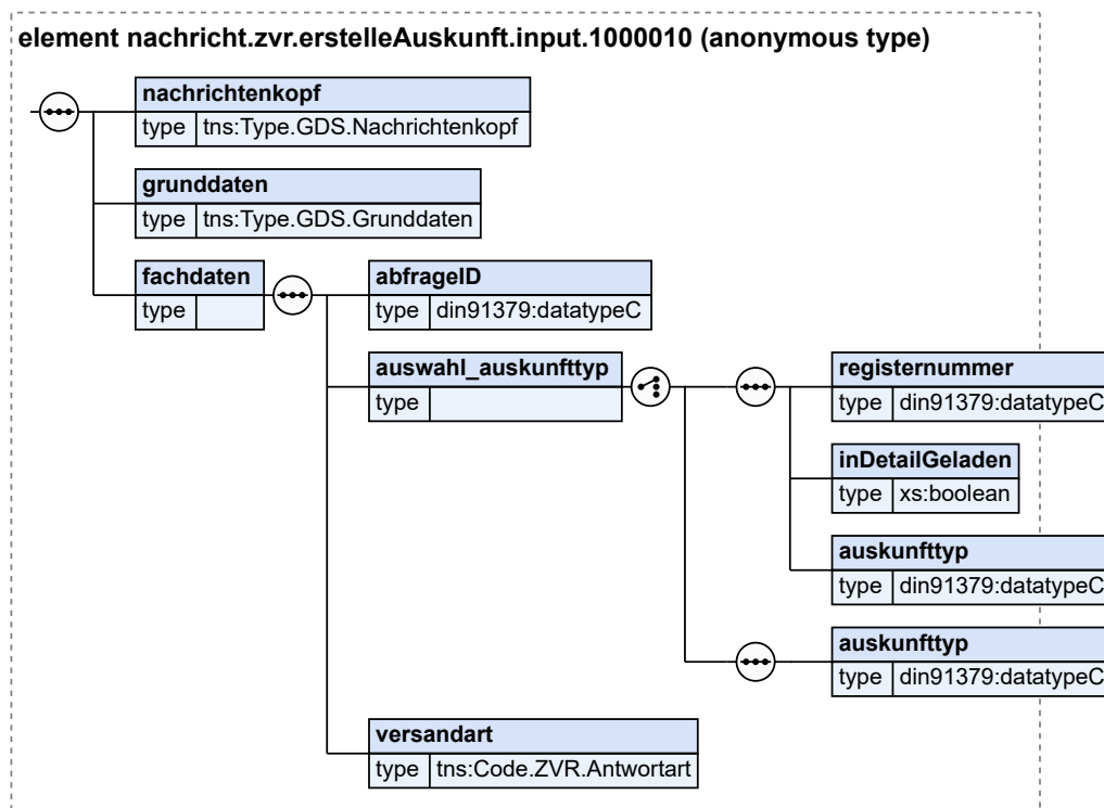
Abbildung 11.11. nachricht.zvr.erstelleAuskunft.input.1000010
