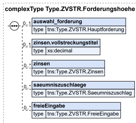
Abbildung 22.13. Type.ZVSTR.Forderungshoehe
