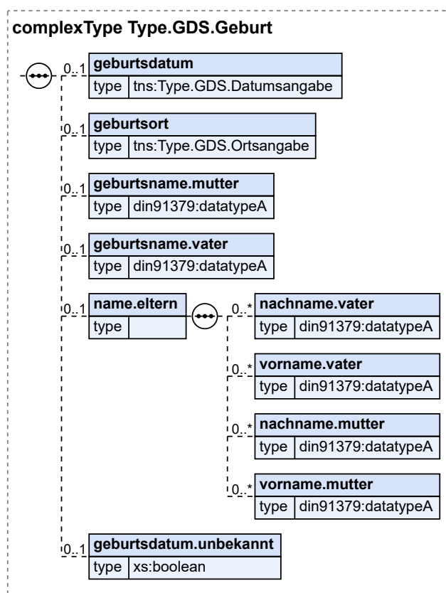
Abbildung 3.16. Type.GDS.Geburt
