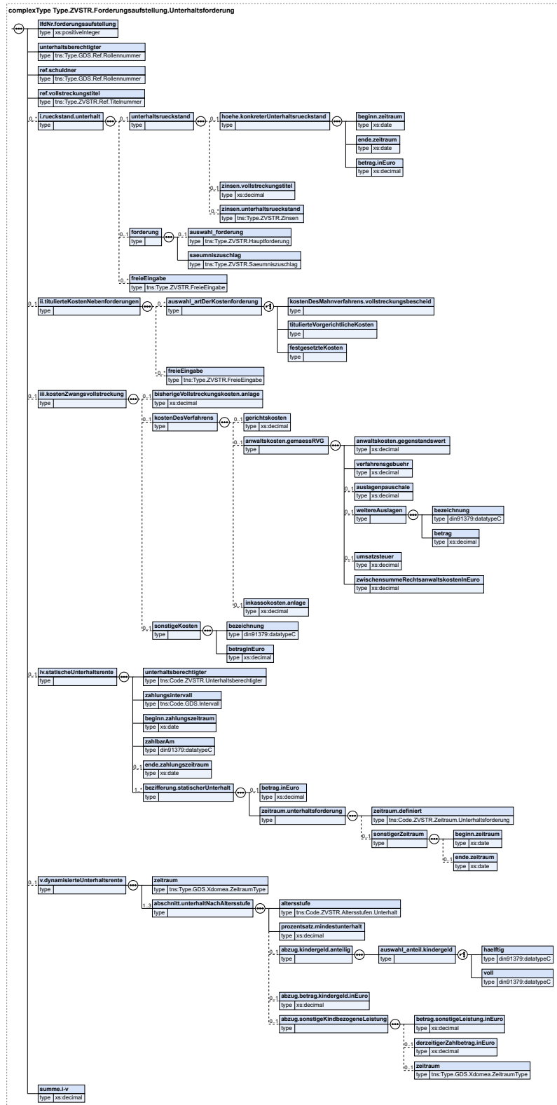
Abbildung 22.11. Type.ZVSTR.Forderungsaufstellung.Unterhaltsforderung
