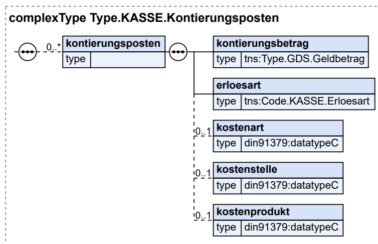
Abbildung 17.35. Type.KASSE.Kontierungsposten
