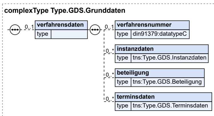
Abbildung 3.4. Type.GDS.Grunddaten
