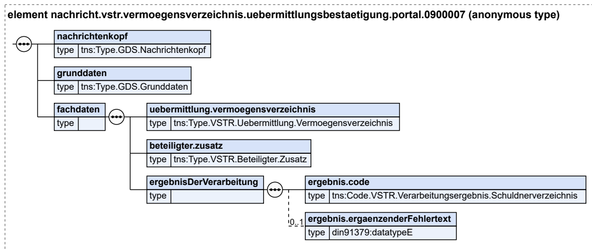
Abbildung 10.24. nachricht.vstr.vermoegensverzeichnis.uebermittlungsbestaetigung.portal.0900007
