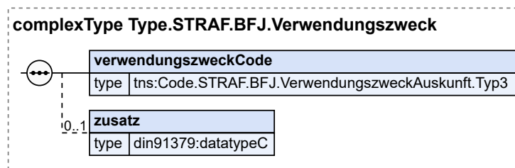
Abbildung 8.89. Type.STRAF.BFJ.Verwendungszweck
