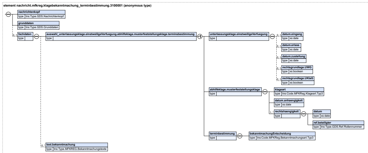
Abbildung 26.17. nachricht.mfkreg.klagebekanntmachung_terminbestimmung.3100001
