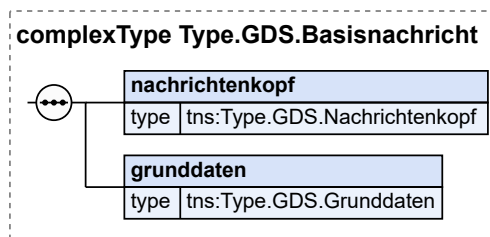
Abbildung 3.10. Type.GDS.Basisnachricht
