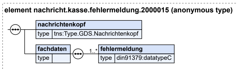
Abbildung 17.59. nachricht.kasse.fehlermeldung.2000015
