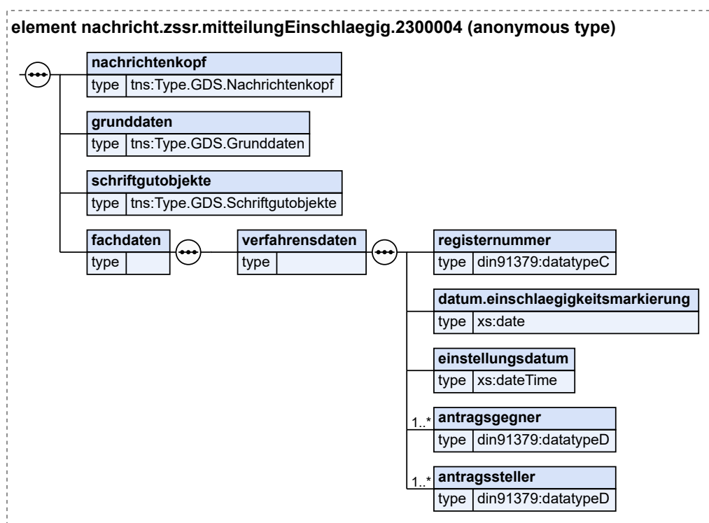
Abbildung 20.7. nachricht.zssr.mitteilungEinschlaegig.2300004
