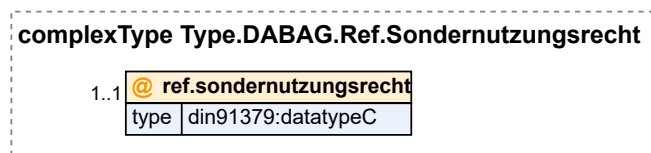
Abbildung 24.53. Type.DABAG.Ref.Sondernutzungsrecht
