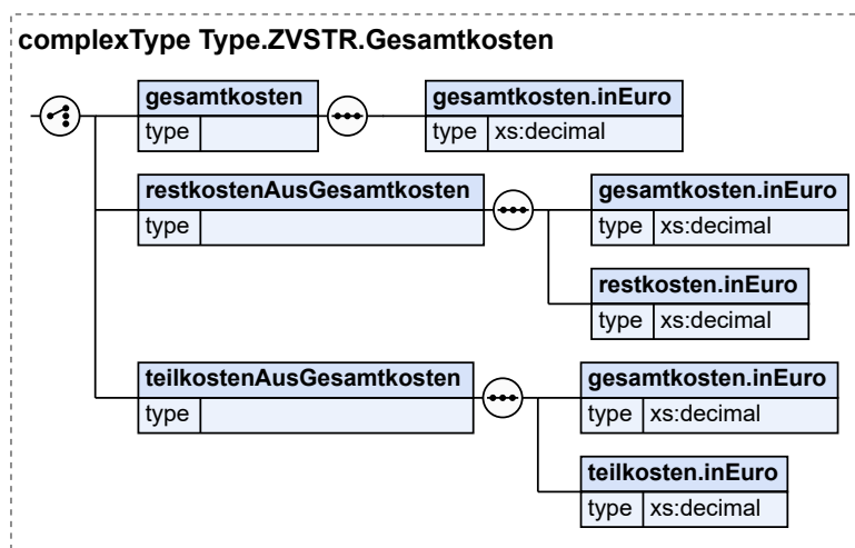
Abbildung 22.15. Type.ZVSTR.Gesamtkosten
