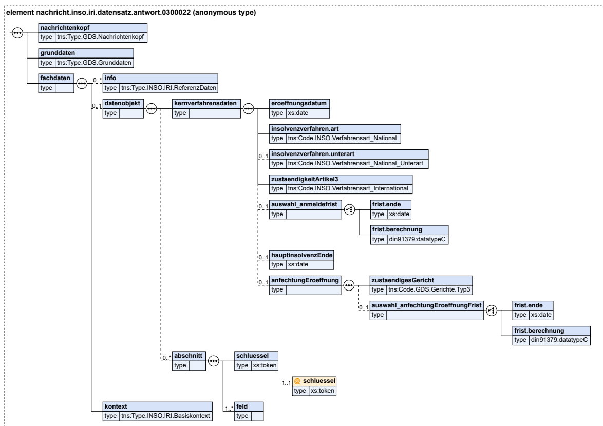
Abbildung 6.43. nachricht.inso.iri.datensatz.antwort.0300022
