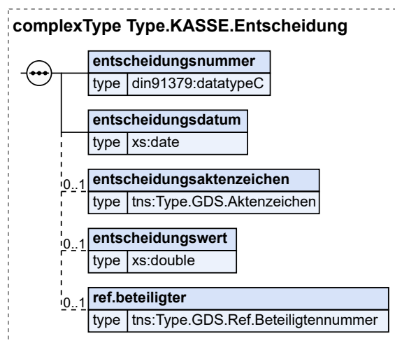
Abbildung 17.32. Type.KASSE.Entscheidung
