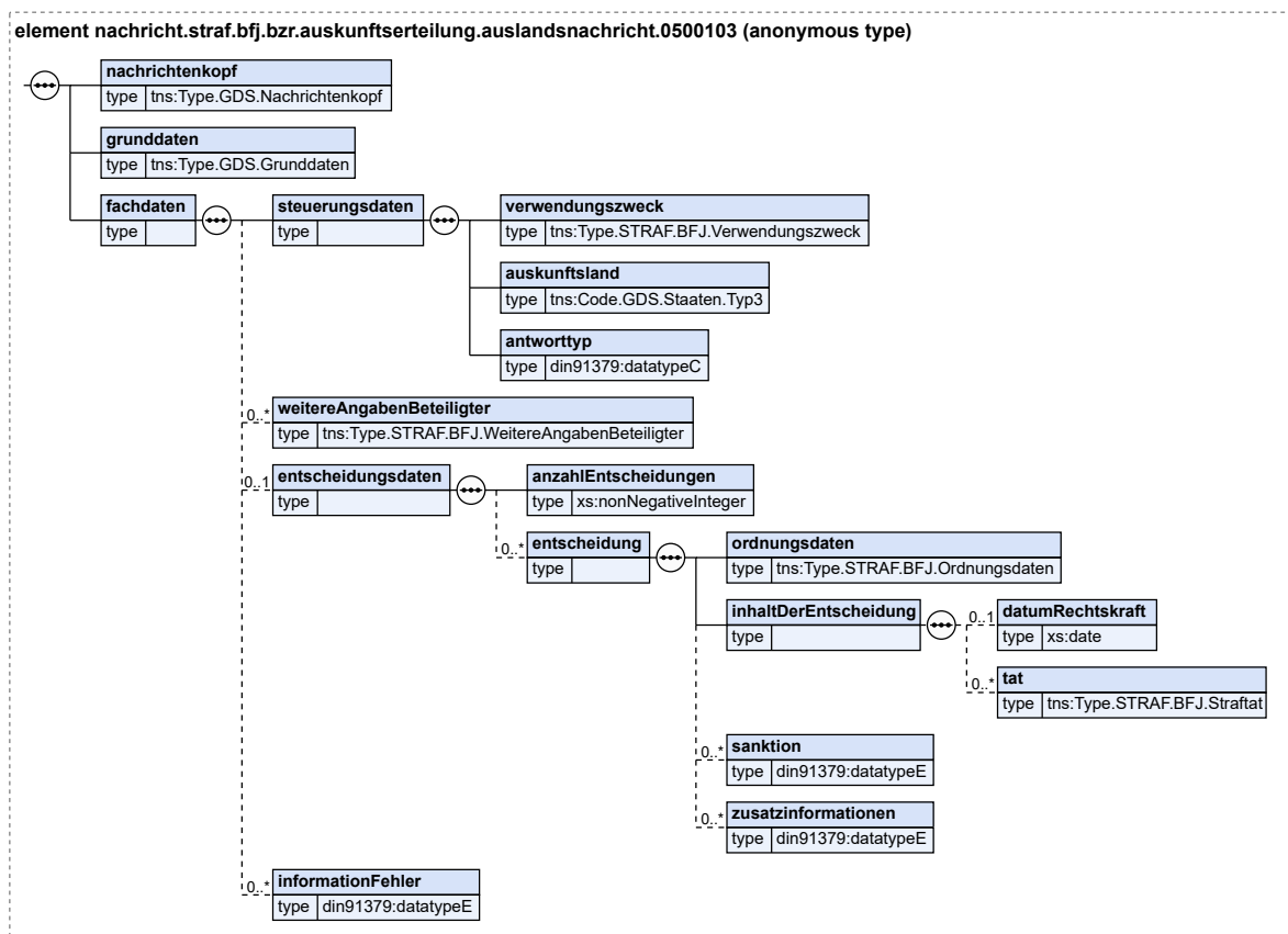
Abbildung 8.93. nachricht.straf.bfj.bzr.auskunftserteilung.auslandsnachricht.0500103
