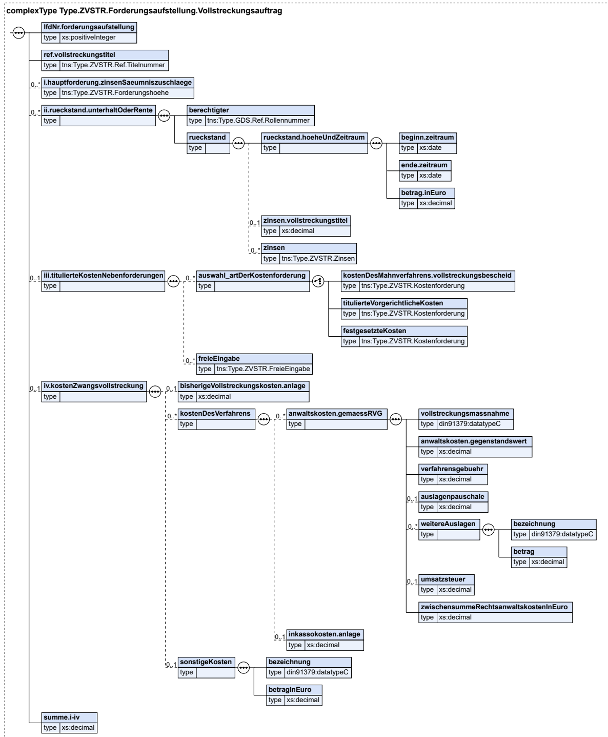
Abbildung 22.12. Type.ZVSTR.Forderungsaufstellung.Vollstreckungsauftrag
