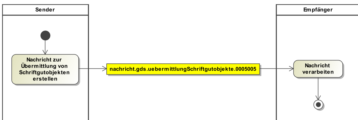
Abbildung 2.2. Kommunikation mittels SGO-Nachricht
