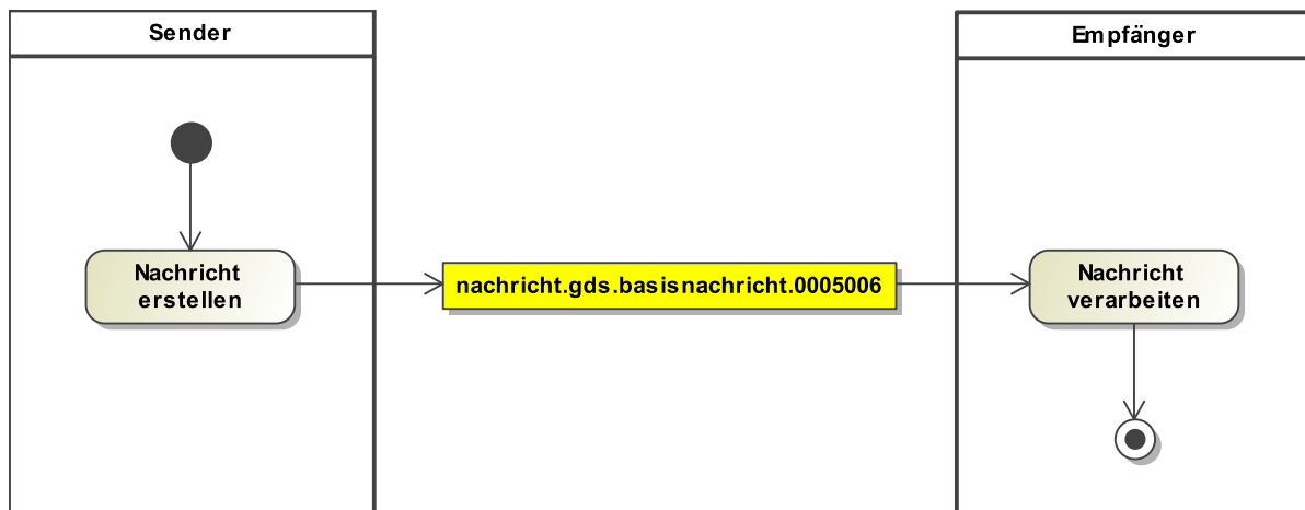
Abbildung 2.1. Kommunikation mittels Basisnachricht
