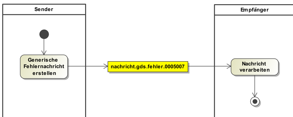
Abbildung 2.3. Kommunikation mittels generischer Fehlernachricht
