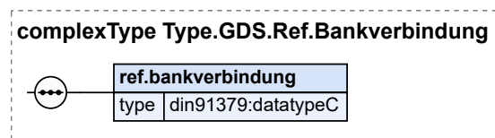
Abbildung 2.34. Type.GDS.Ref.Bankverbindung
