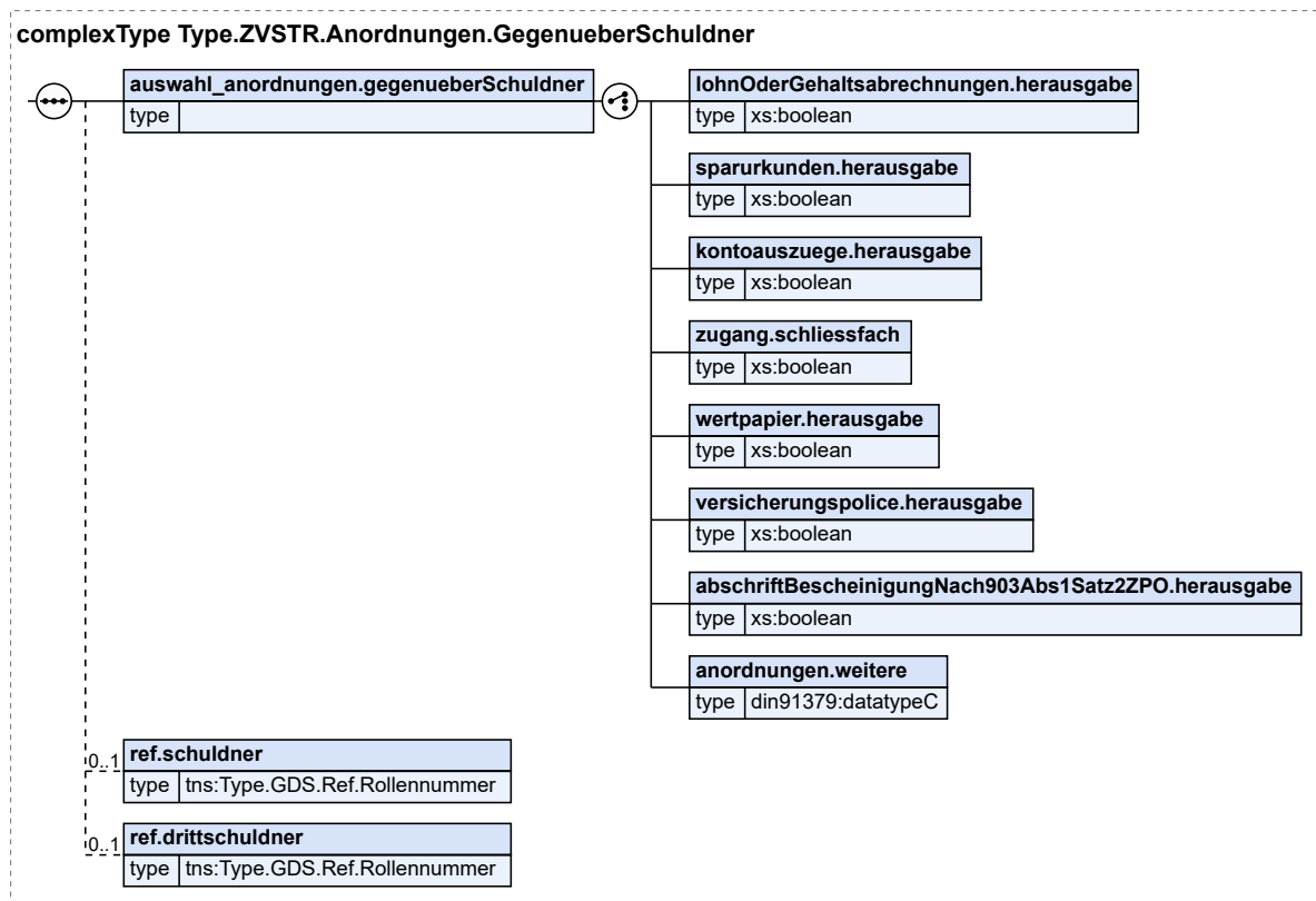
Abbildung 3.5. Type.ZVSTR.Anordnungen.GegenueberSchuldner
