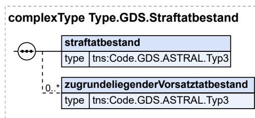
Abbildung 2.41. Type.GDS.Straftatbestand
