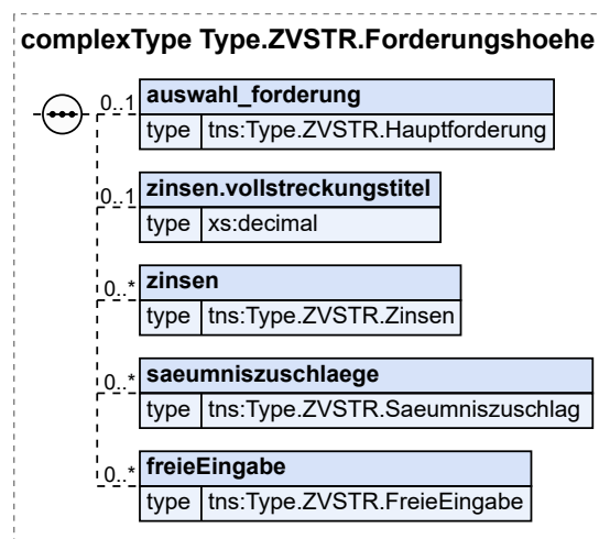
Abbildung 3.13. Type.ZVSTR.Forderungshoehe
