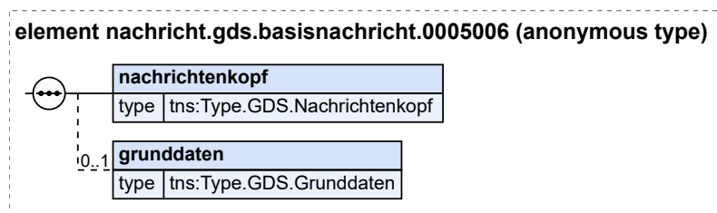
Abbildung 2.57. nachricht.gds.basisnachricht.0005006
