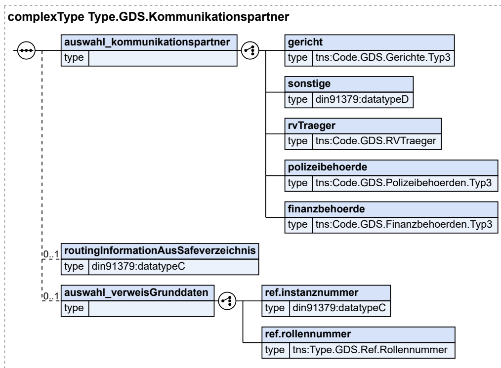
Abbildung 2.25. Type.GDS.Kommunikationspartner
