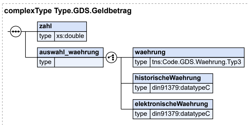
Abbildung 2.20. Type.GDS.Geldbetrag
