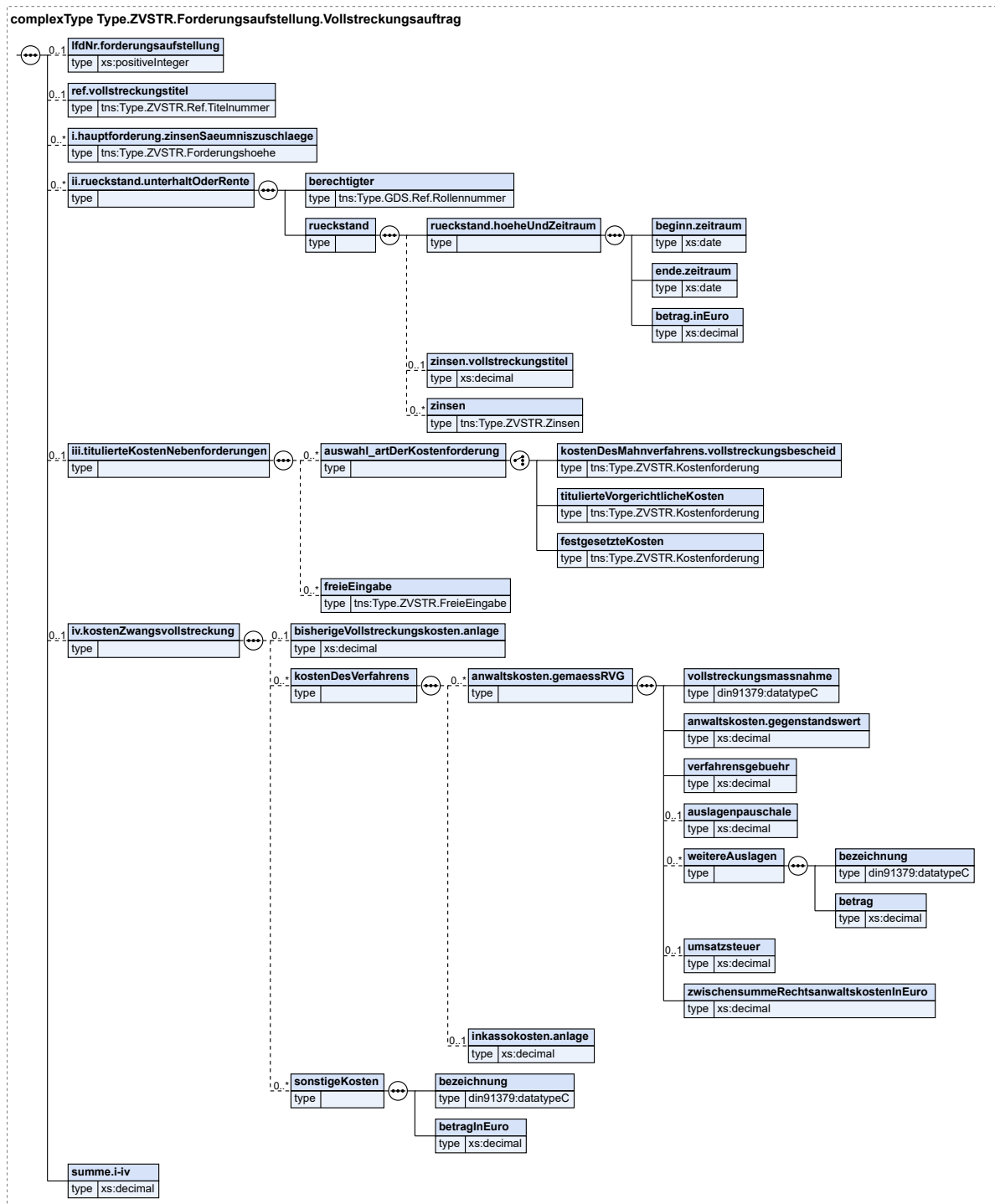
Abbildung 3.12. Type.ZVSTR.Forderungsaufstellung.Vollstreckungsauftrag
