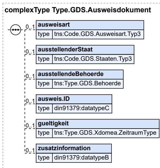
Abbildung 2.8. Type.GDS.Ausweisdokument
