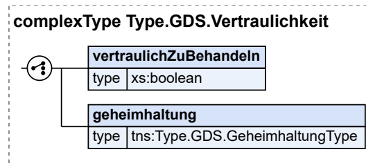
Abbildung 2.47. Type.GDS.Vertraulichkeit
