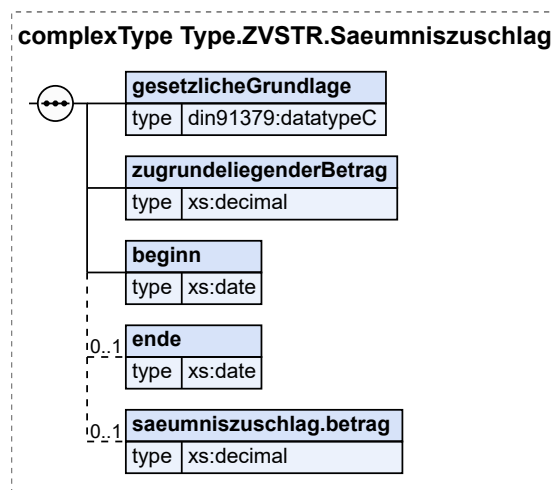
Abbildung 3.20. Type.ZVSTR.Saeumniszuschlag
