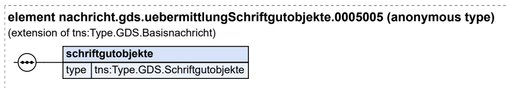
Abbildung 2.56. nachricht.gds.uebermittlungSchriftgutobjekte.0005005
