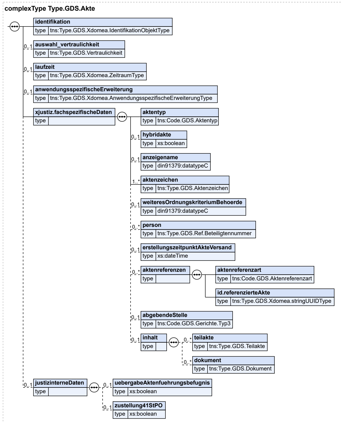
Abbildung 2.5. Type.GDS.Akte
