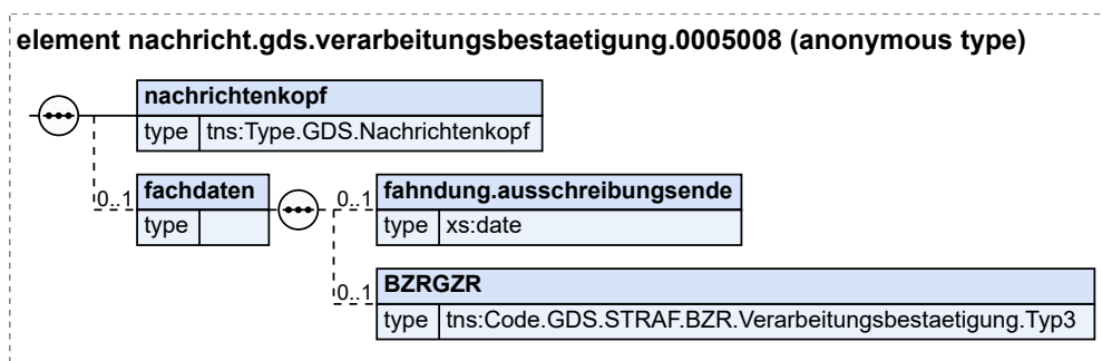
Abbildung 2.59. nachricht.gds.verarbeitungsbestaetigung.0005008
