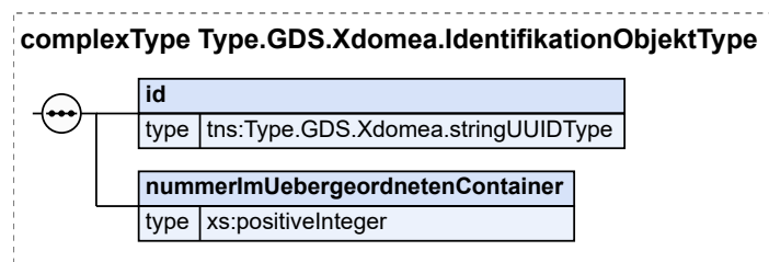
Abbildung 2.51. Type.GDS.Xdomea.IdentifikationObjektType
