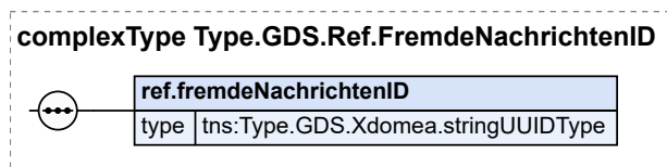
Abbildung 2.36. Type.GDS.Ref.FremdeNachrichtenID
