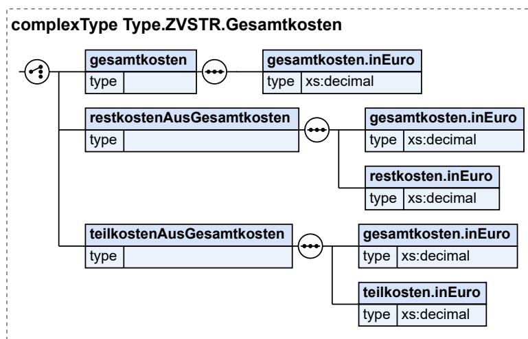
Abbildung 3.15. Type.ZVSTR.Gesamtkosten
