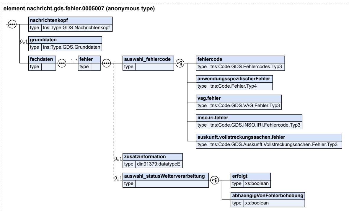
Abbildung 2.58. nachricht.gds.fehler.0005007
