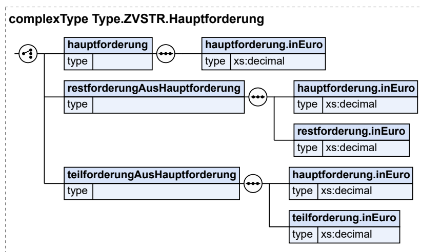
Abbildung 3.16. Type.ZVSTR.Hauptforderung
