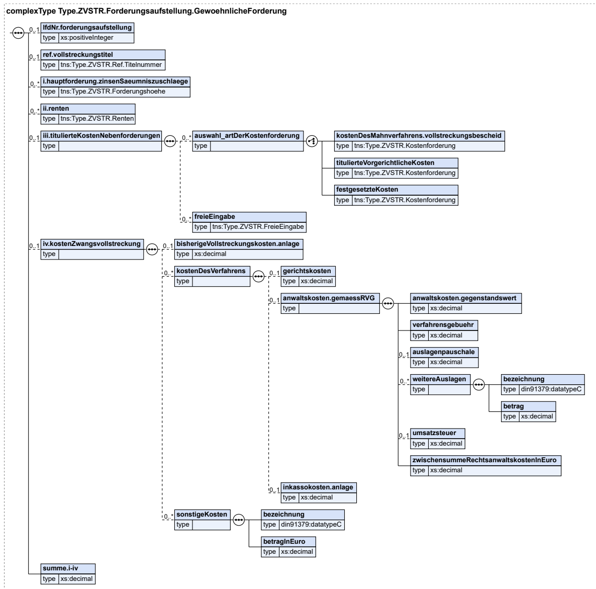
Abbildung 3.10. Type.ZVSTR.Forderungsaufstellung.GewoehnlicheForderung
