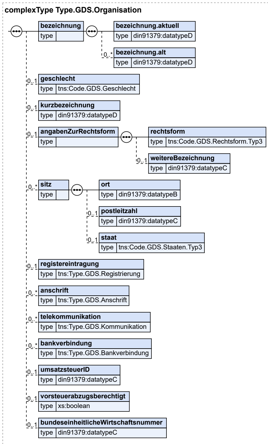
Abbildung 2.31. Type.GDS.Organisation
