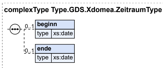
Abbildung 2.52. Type.GDS.Xdomea.ZeitraumType
