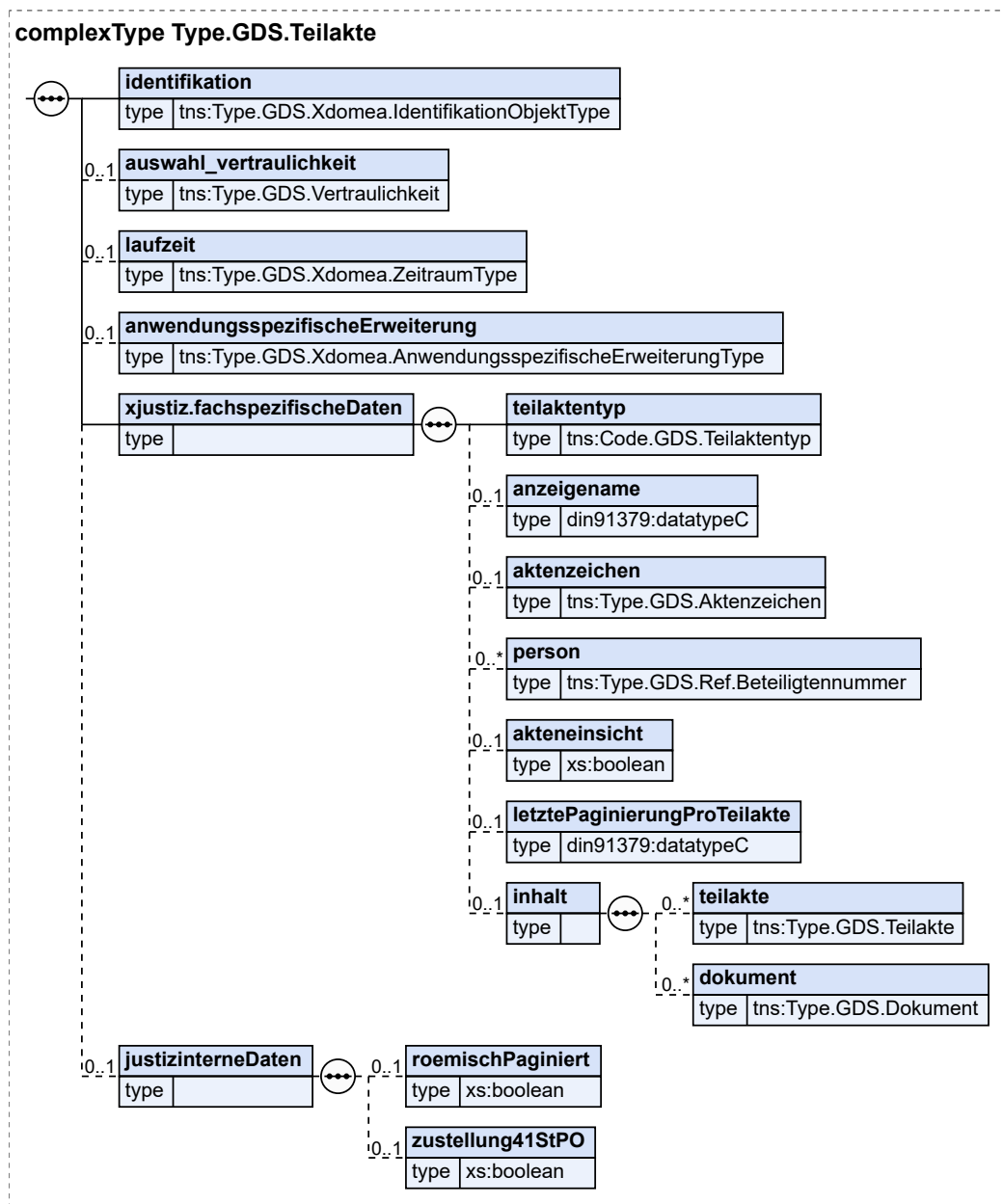
Abbildung 2.43. Type.GDS.Teilakte
