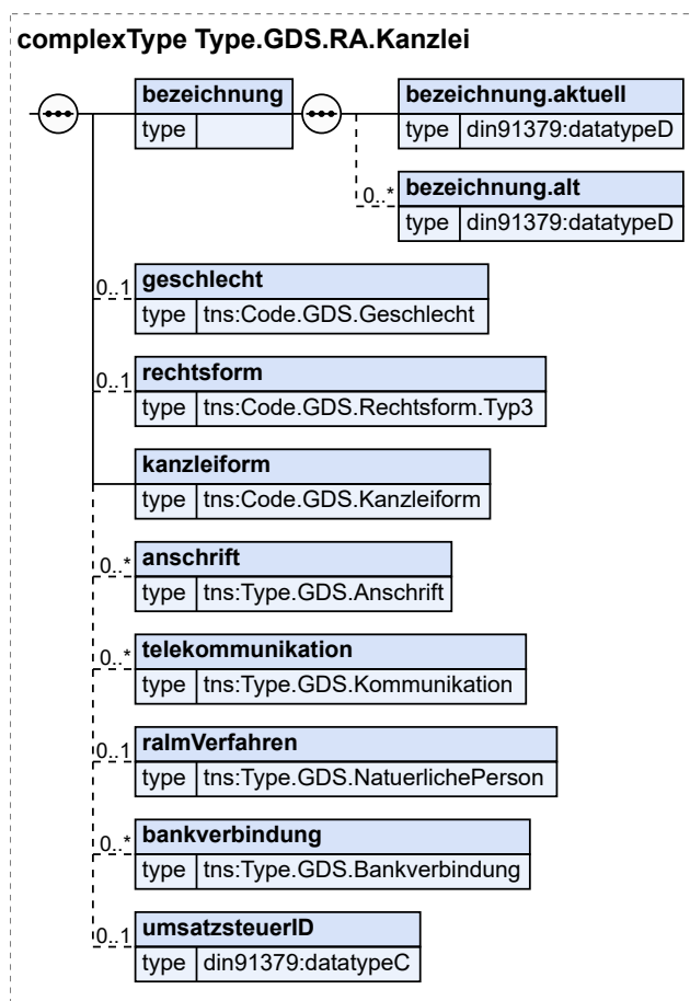
Abbildung 2.33. Type.GDS.RA.Kanzlei
