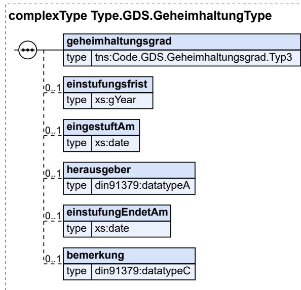
Abbildung 2.18. Type.GDS.GeheimhaltungType
