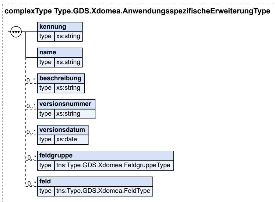
Abbildung 2.48. Type.GDS.Xdomea.AnwendungsspezifischeErweiterungType
