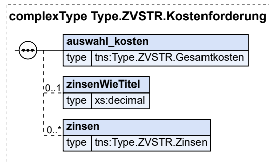
Abbildung 3.17. Type.ZVSTR.Kostenforderung
