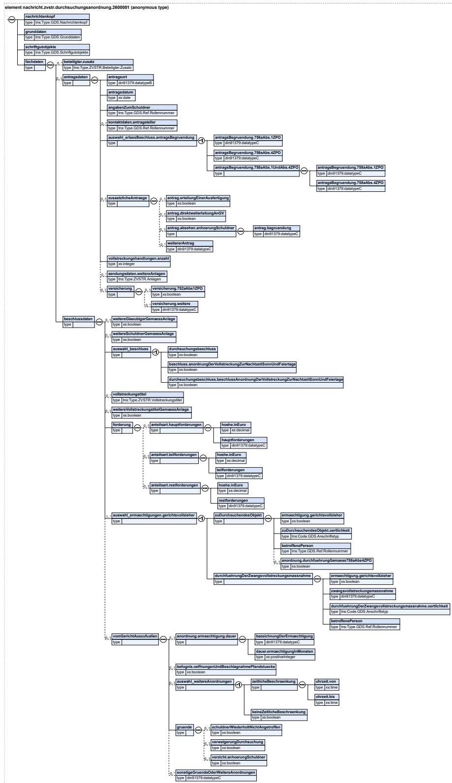
Abbildung 3.23. nachricht.zvstr.durchsuchungsanordnung.2600001
