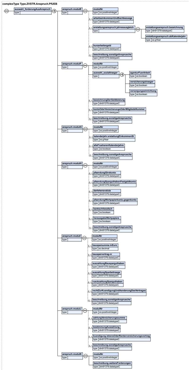
Abbildung 3.6. Type.ZVSTR.Anspruch.PFUEB
