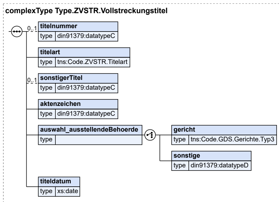
Abbildung 3.21. Type.ZVSTR.Vollstreckungstitel
