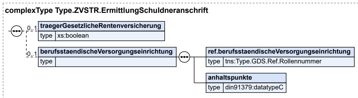
Abbildung 3.9. Type.ZVSTR.ErmittlungSchuldneranschrift
