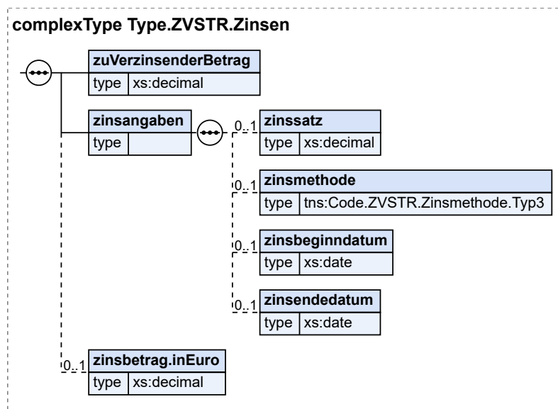
Abbildung 3.22. Type.ZVSTR.Zinsen
