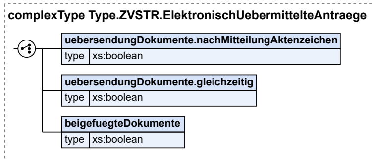
Abbildung 3.8. Type.ZVSTR.ElektronischUebermittelteAntraege
