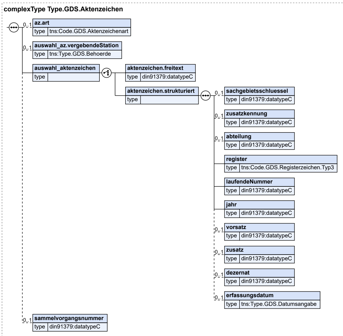
Abbildung 2.6. Type.GDS.Aktenzeichen
