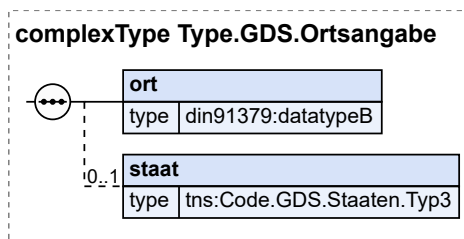
Abbildung 2.32. Type.GDS.Ortsangabe
