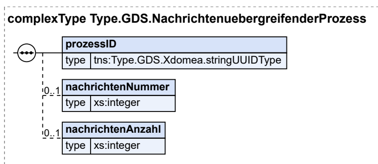
Abbildung 2.28. Type.GDS.NachrichtenebergreifenderProzess
