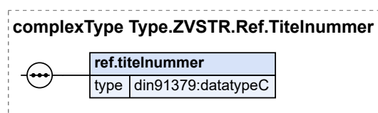
Abbildung 3.19. Type.ZVSTR.Ref.Titelnummer
