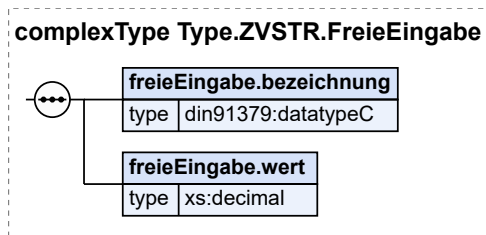
Abbildung 3.14. Type.ZVSTR.FreieEingabe
