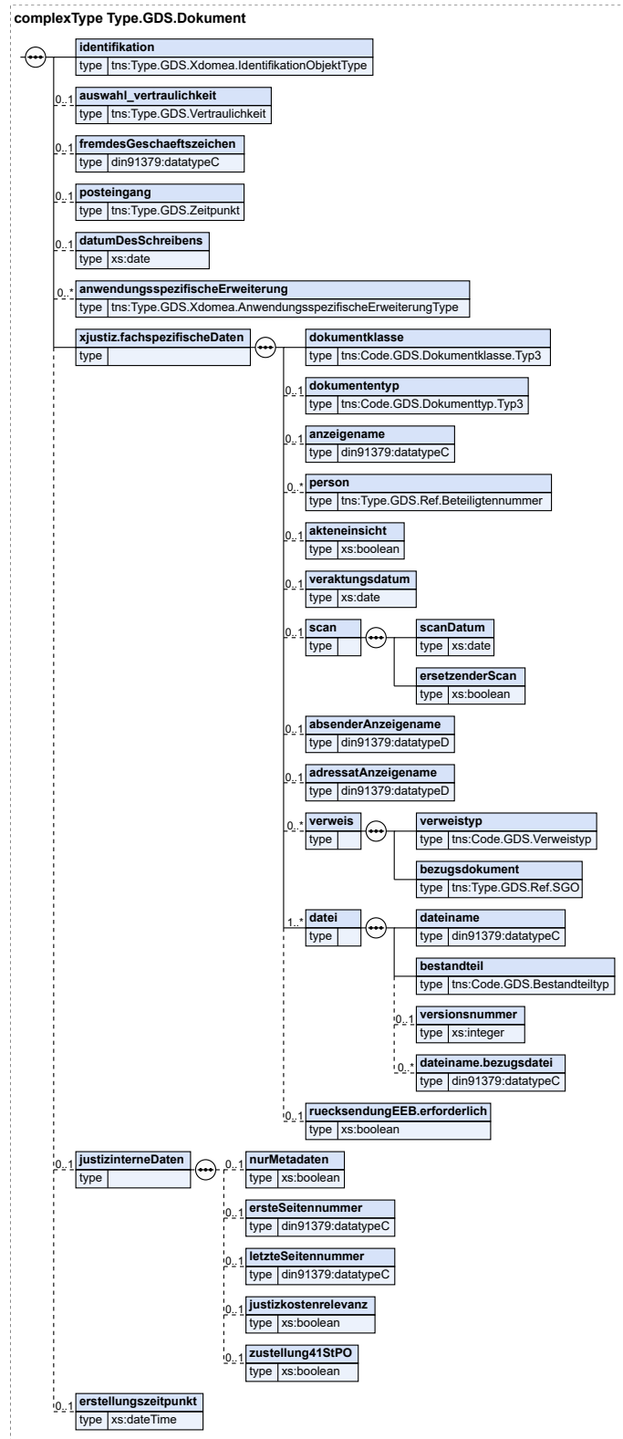
Abbildung 2.16. Type.GDS.Dokument
