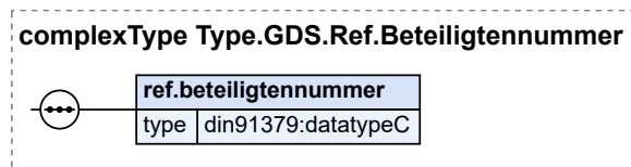
Abbildung 2.35. Type.GDS.Ref.Beteiligtennummer
