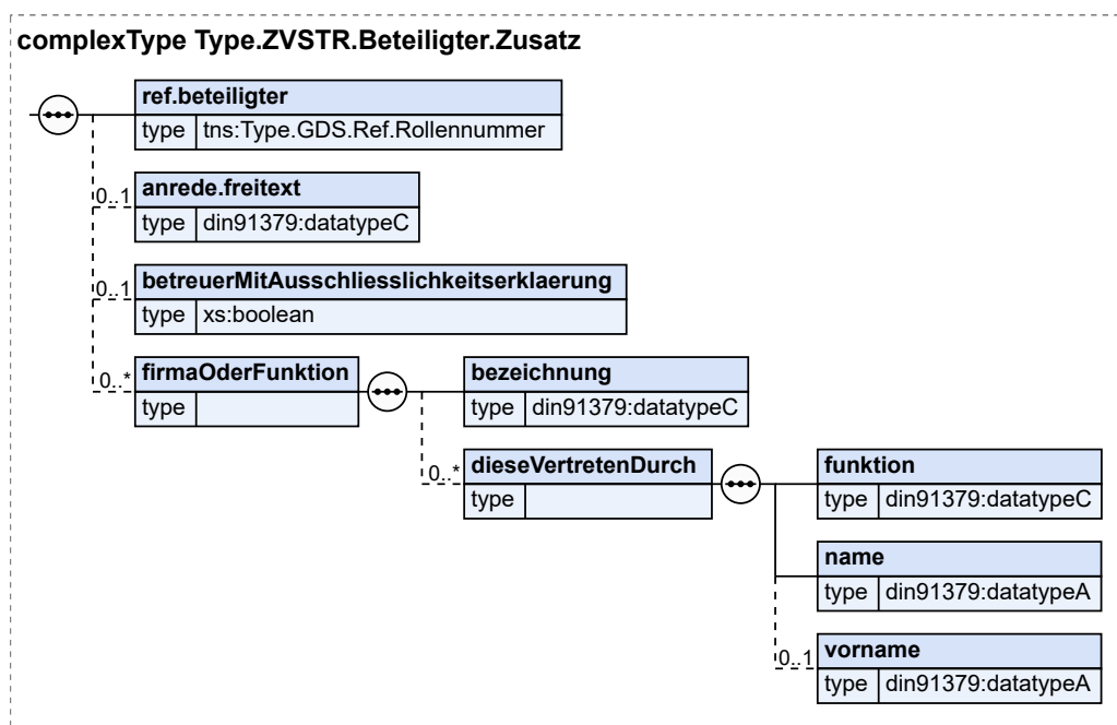
Abbildung 3.7. Type.ZVSTR.Beteiligter.Zusatz
