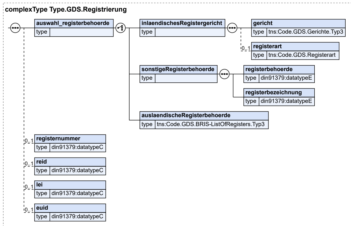
Abbildung 2.39. Type.GDS.Registrierung
